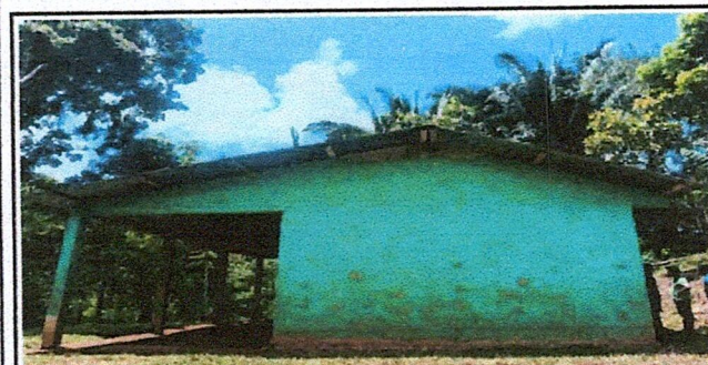
Fotografía 5: por falta de agua entubada en la comunidad se necesita un almacen de agua y una pila plastica, asi como la base de concreto para el almacenamiento del agua.
