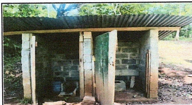
Fotografía 3: baños en muy mal estado se requiere subir altura, repello, cambio de lamina y costanera de metal asi como puertas de metal y cambio de letrinas.
